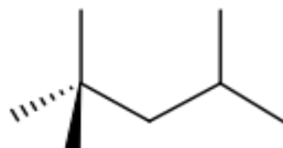
Iso-octano
